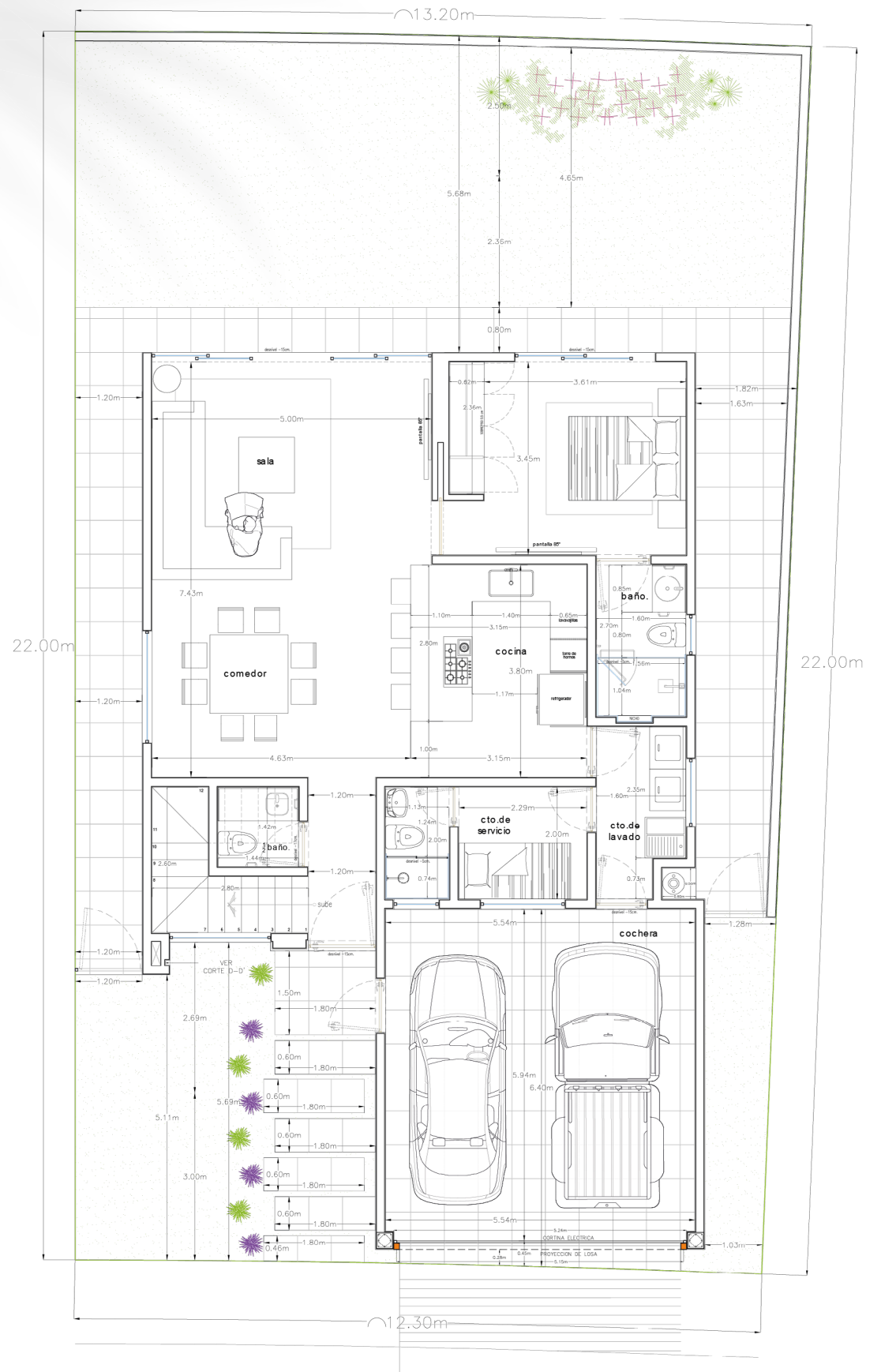
PLANTA BAJA
