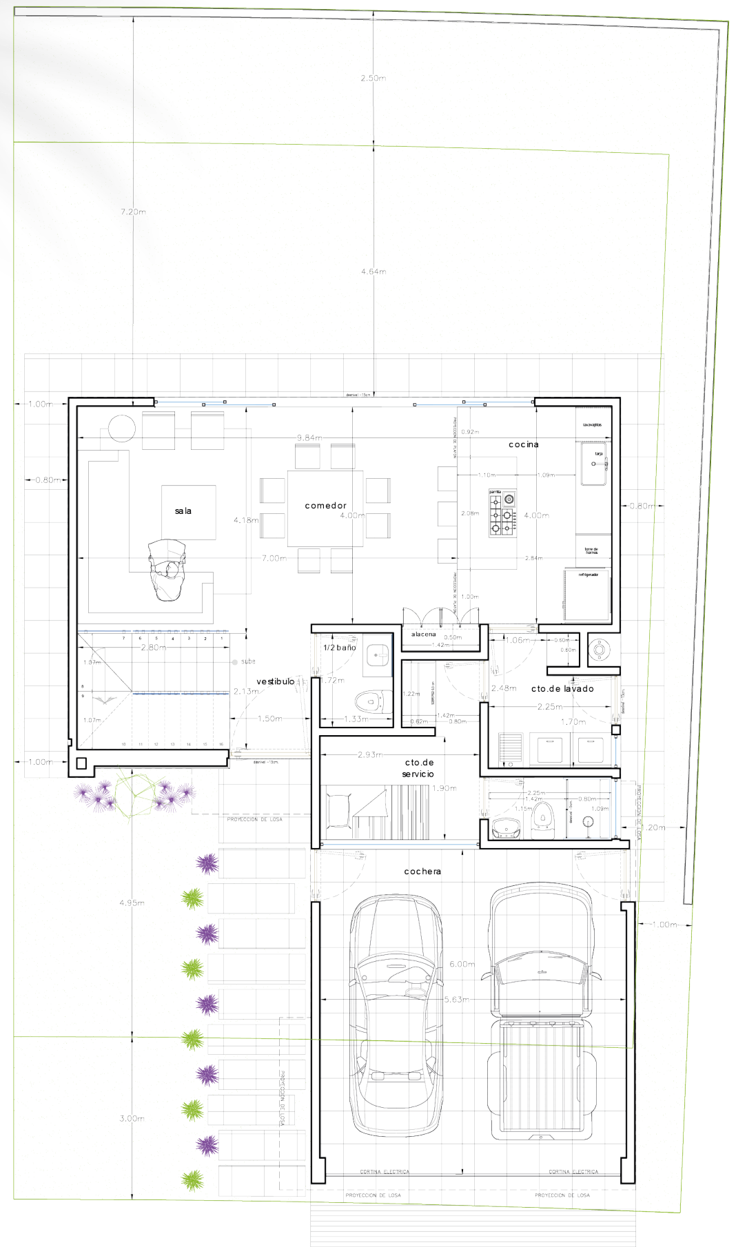
PLANTA BAJA
