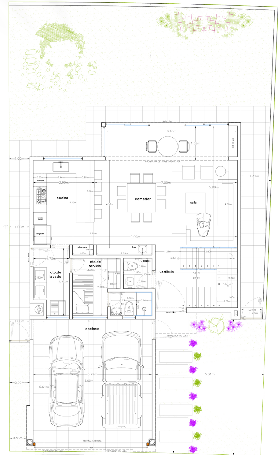
PLANTA BAJA
